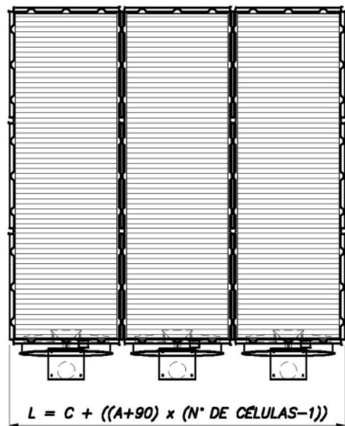
PLANTA CÁLCULO DO COMPRIMENTO (L) P/ TORRES MULTICELULARES
